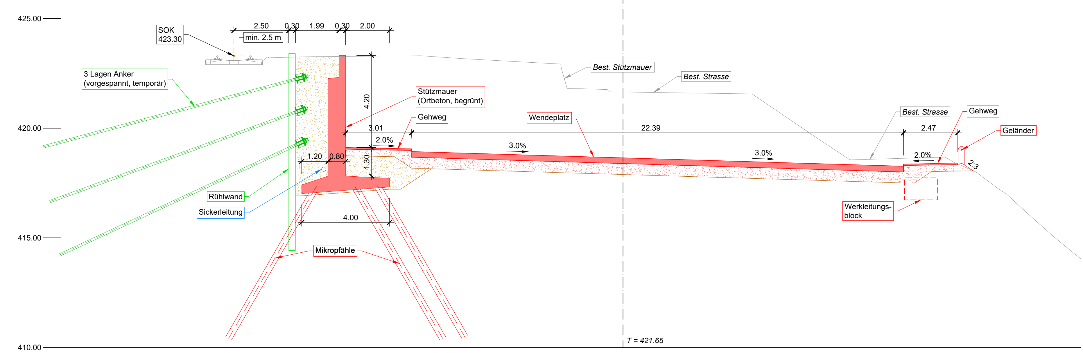
QUERPROFIL m 120, 1:100
