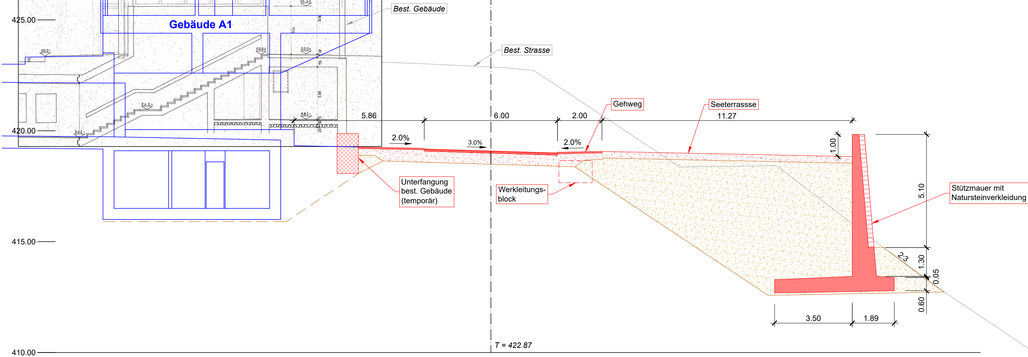
QUERPROFIL m 150, 1:100
