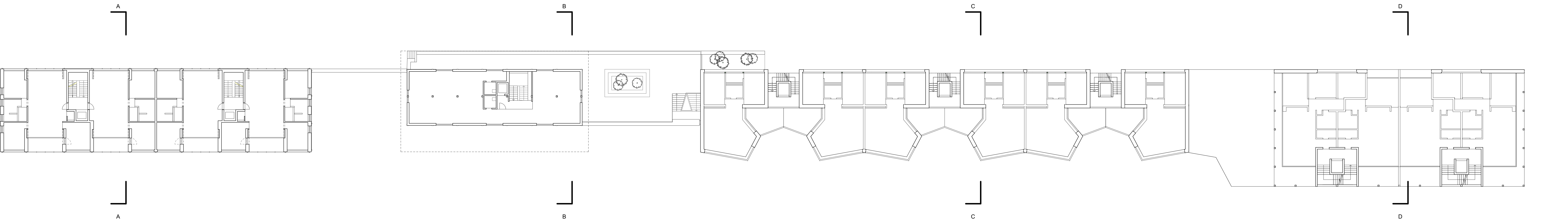
Grundriss 2.Obergeschoss M 1:200
